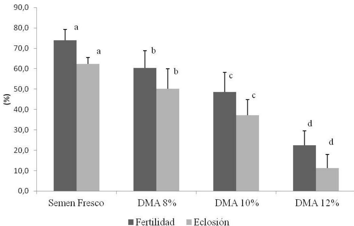
Figura 1. Tasas de fertilidad y de eclosión de bocachico Prochilodus magdalenae inseminado con semen fresco y criopreservado-descongelado con DMA a diferentes concentraciones. Entre tratamientos, valores con letras distintas son significativamente diferentes ( P < 0,05 ).
