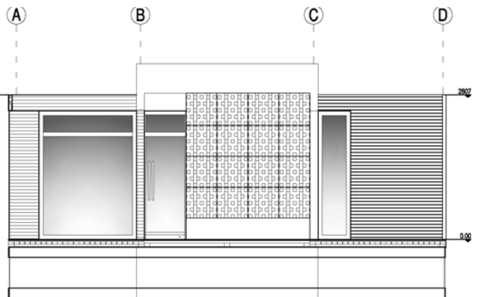
Corte B-B
