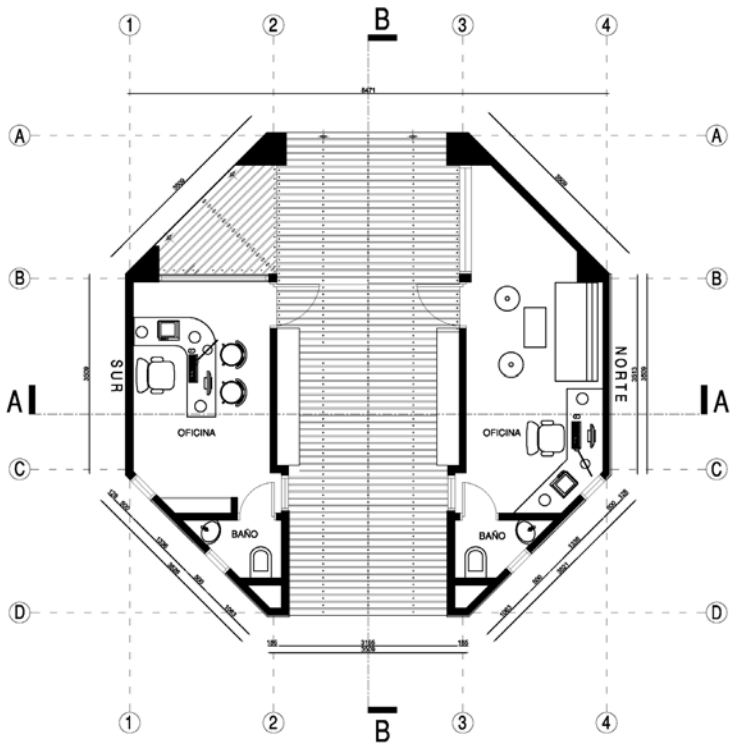
Planta Arquitectura
