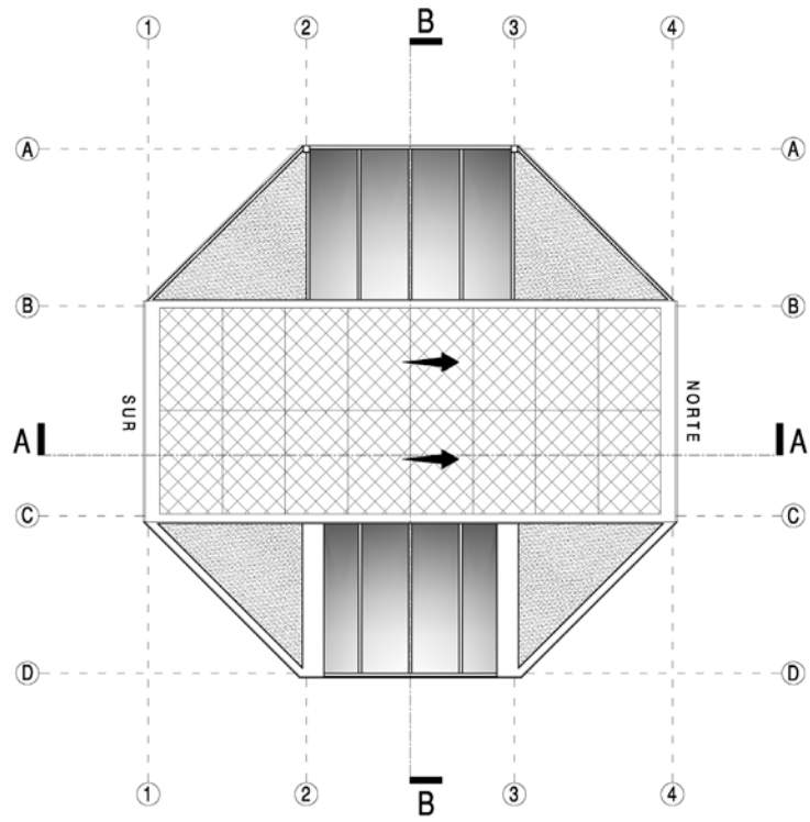
Planta Cubierta
