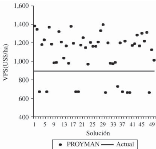
Figura 1. Comparación Valor Potencial del Suelo en soluciones PROYMAN versus solución Actual . Comparison Bare Land Value in solutions PROYMAN versus solution Present .
