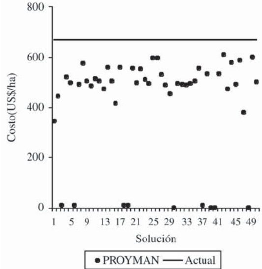
Figura 2. Comparación Costo de Establecimiento en soluciones PROYMAN versus solución Actual . Comparison Cost of Establishment in solutions PROYMAN versus solution Present .
