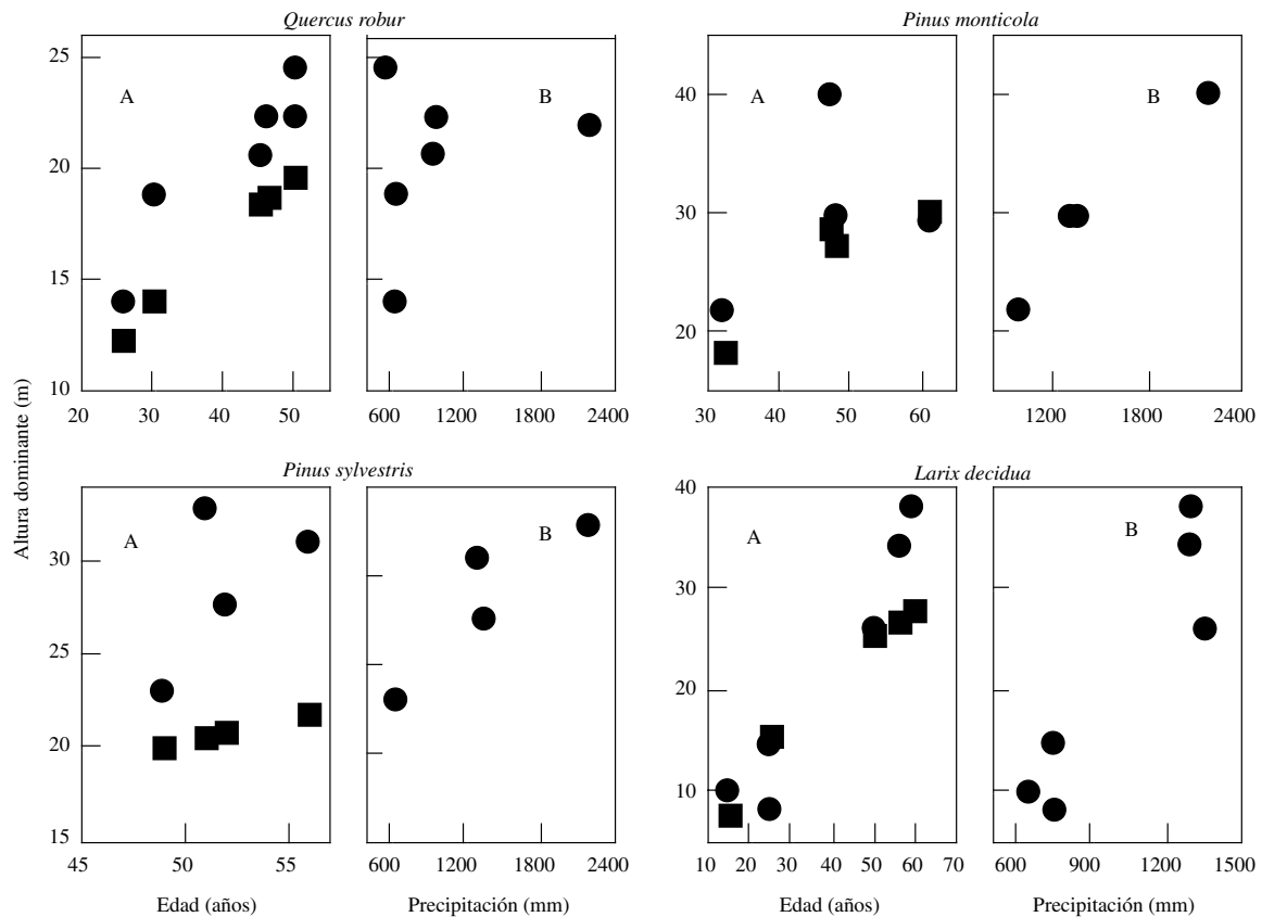
Figura 1. Alturas dominantes de diferentes especies: A) medidas en Patagonia (círculos) y en el lugar de origen según Schober (1987) (cuadrados) para Quercus robur , Pinus sylvestris y Larix decidua , y según Curtis et al. (1990) para Pinus monticola ; B) en relación a las precipitaciones anuales.
