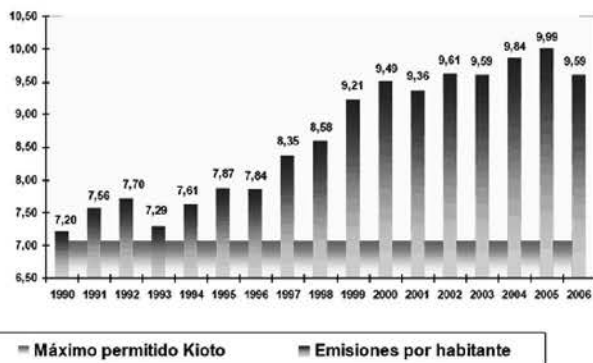
Gráfico de emisión de CO2. Caso de España entre 1990-2006.
